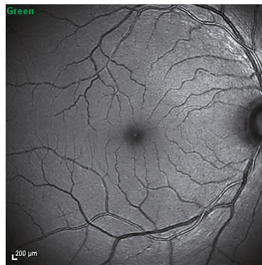
Green : 518 nm
