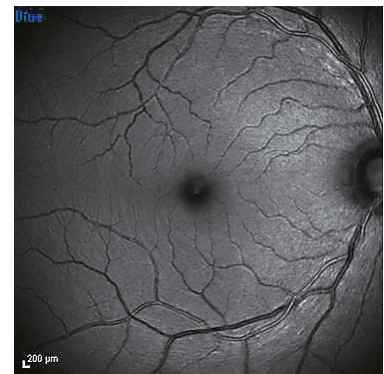
Blue : 488 nm
