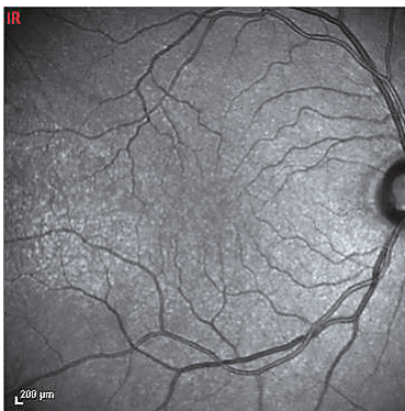
Infrared : 815 nm
